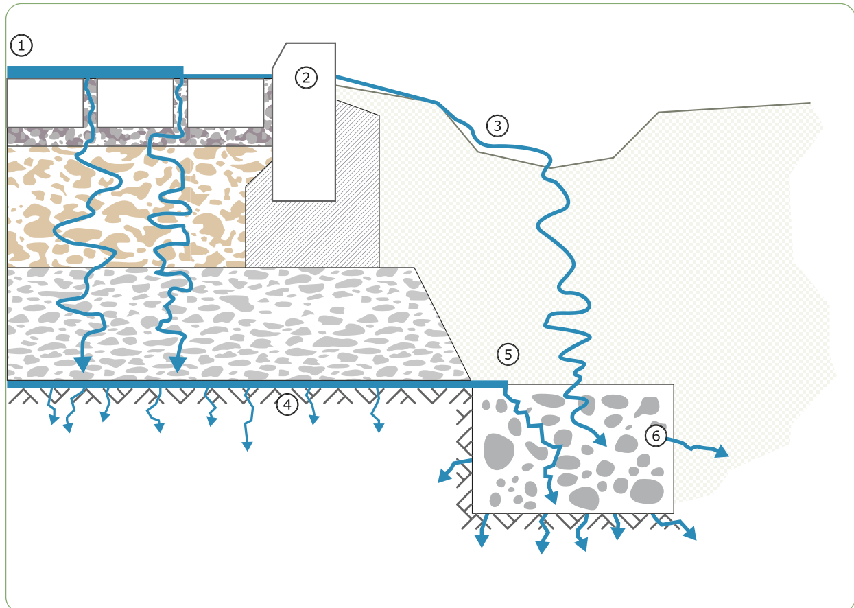
Abbildung 11: Schematische Darstellung einer versickerungsfähigen Pflasterfläche bei gering durchlässigem Untergrund ( 3 \cdot 10^{-6} \text{ m/s} \leq k_i Untergrund 3 \cdot 10^{-5} )
