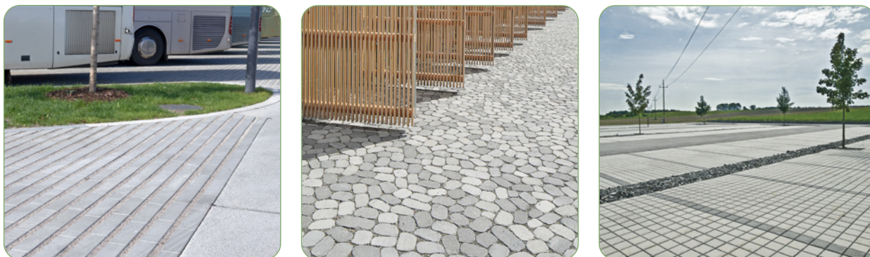
Abbildung 4: Betonstein mit aufgeweiteter Sickerfuge und kapillarer Grünfugenfüllung
